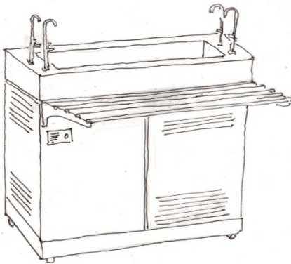
Σκαρίφημα της προτεινόμενης μορφής του ψύκτη νερού και δείγμα του τύπου της βρύσης.
