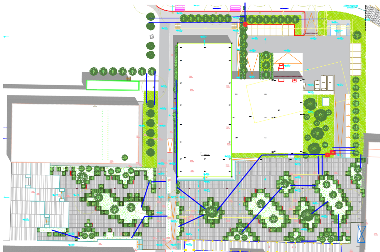
Εικόνα 3β – Τμήμα Β, αποτύπωσης διαμόρφωσης δικτύου άρδευσης
