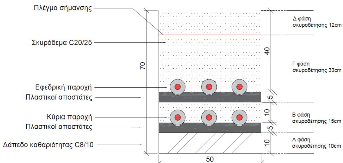
ΣΧ. 2. ΤΟΜΗ ΧΑΝΔΑΚΑ
