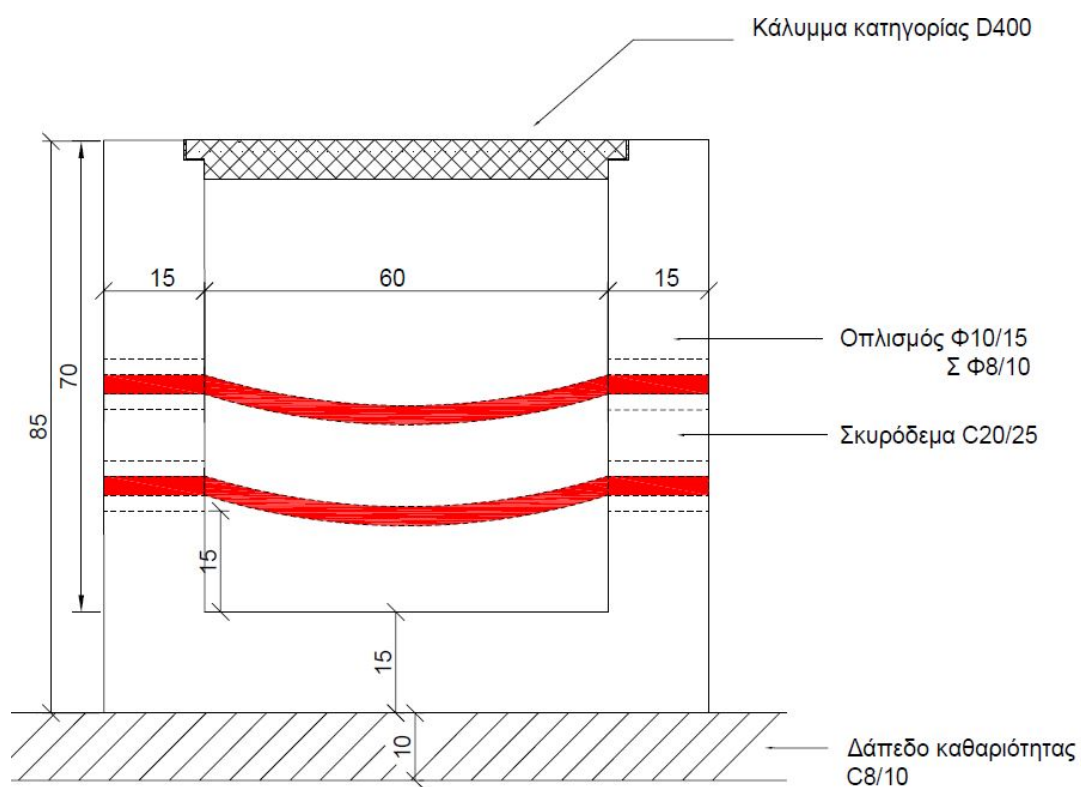
ΣΧ. 3 ΤΟΜΗ ΦΡΕΑΤΙΟΥ
