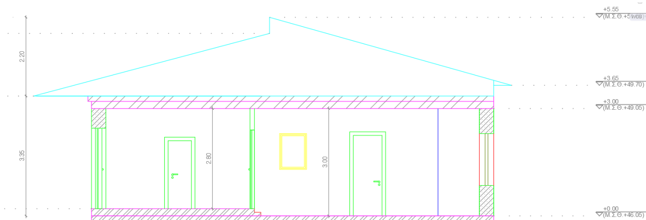
Σκαρίφημα 4: Τομή 2 του κτιρίου Κ.1.1.2.
